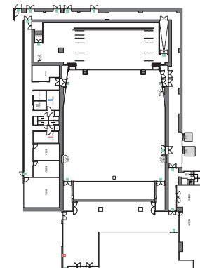
図面(フラット)
