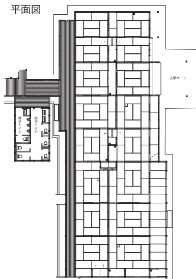
平面図
