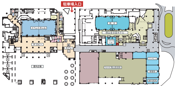
1F 平面図
